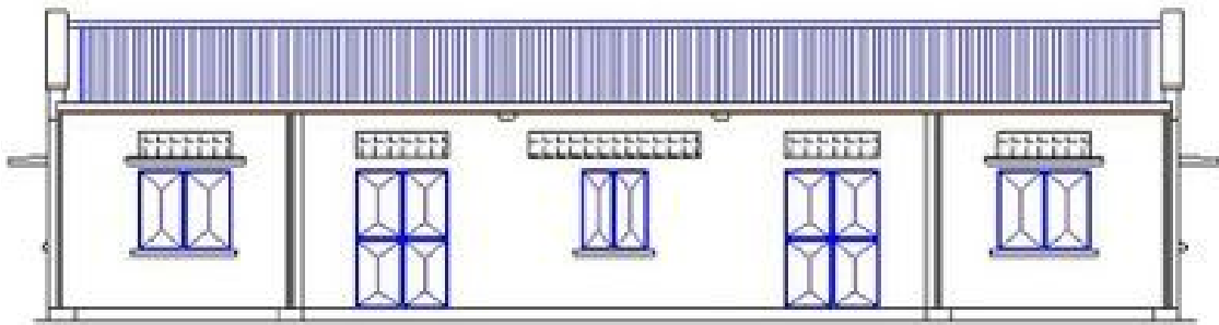
FACADE PRICIPALE éch. : 1/100
